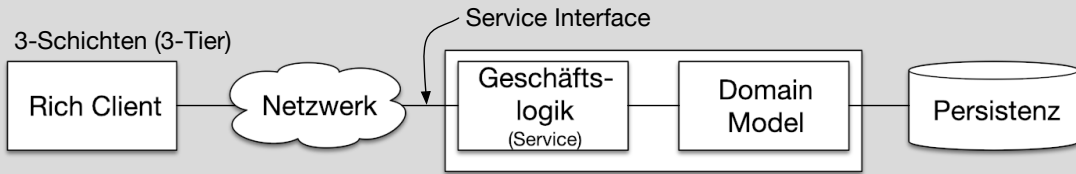
N-Tier
